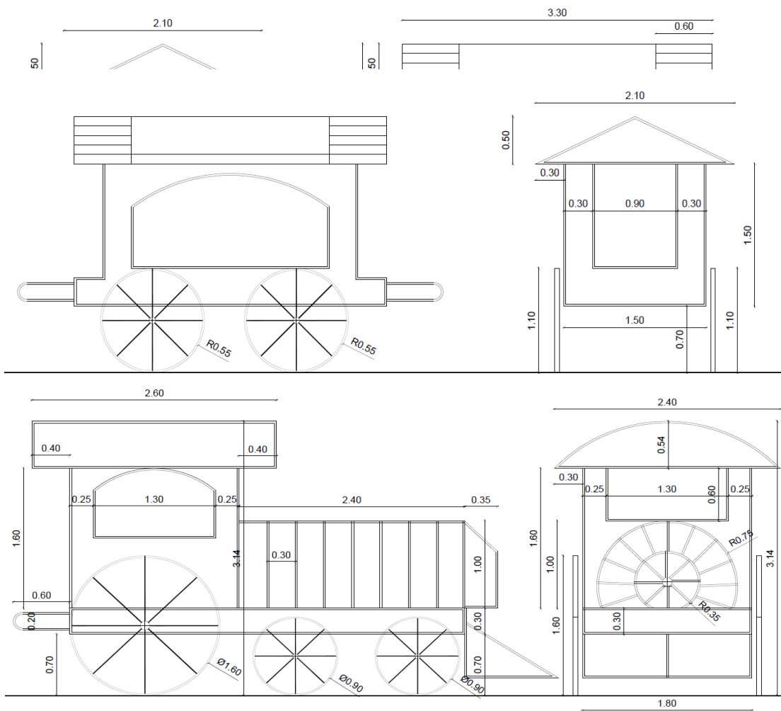
Σχέδιο 3: Χριστουγεννιάτικες μεταλλικό τρενάκι
